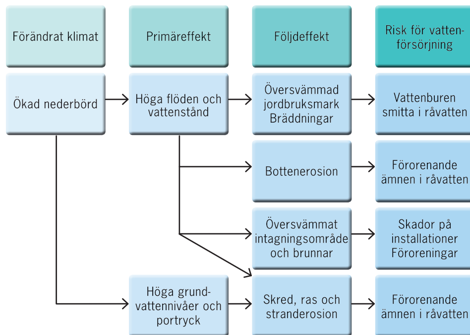
Figur 18. Exempel på effekter av ett förändrat klimat på dricksvattenförsörjning.
